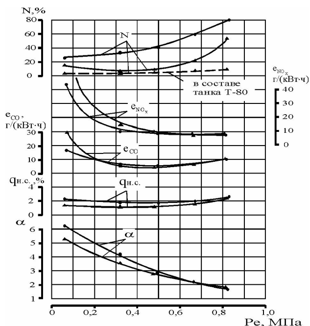
Рис. 1. Нагрузочные характеристики при номинальной частоте вращения коленчатого вала
