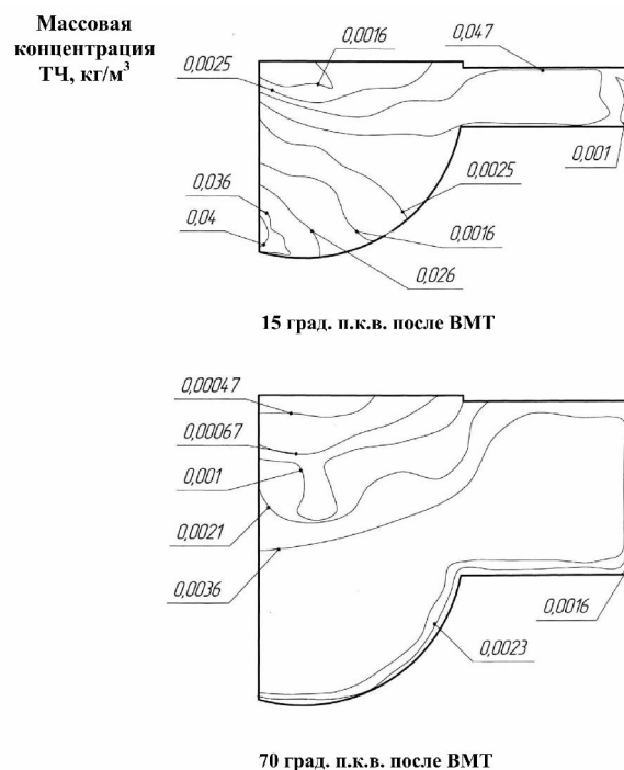
Рис. 8. Изменение массовой концентрации ТЧ в цилиндре дизеля в зависимости от угла поворота коленчатого вала (режим с N_e = 18,4 кВт при n = 1800 мин -1 )
