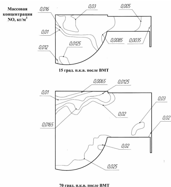
Рис. 7. Изменение массовой концентрации NO в цилиндре дизеля, в зависимости от угла поворота коленчатого вала (режим с N_e = 18,4 кВт при n = 1800 мин -1 )
