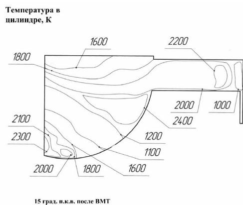
Рис. 6. Распределение температуры в цилиндре дизеля в процессе горения топливовоздушной смеси (режим с N_e = 18,4 кВт, при n = 1800 мин -1 )
