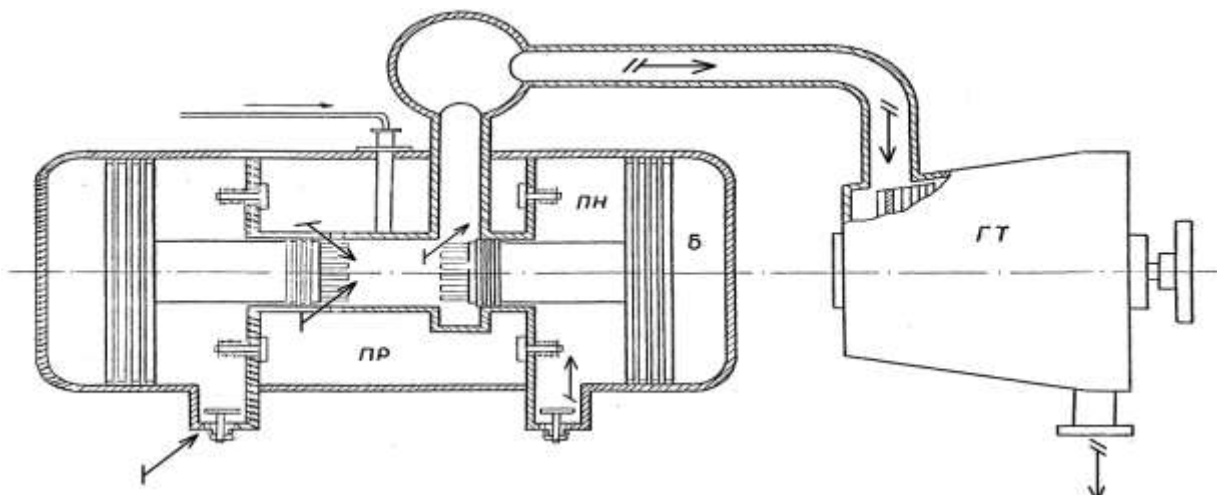
Рис.2. Вільнопоршневий двигун - генератор газу:
