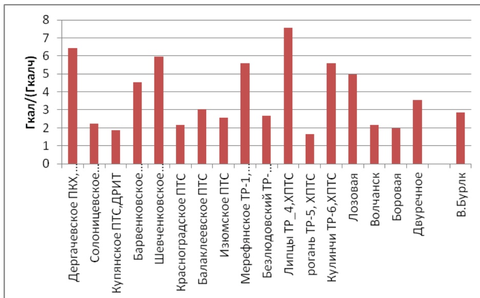
Рис.4. Отношение установленной мощности оборудования к присоединенной нагрузке, Гкал/ч/(Гкал/ч)
