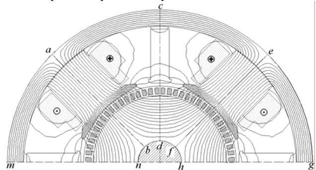
Рис. 3. Расчетная модель и картина магнитного поля МПТ с беззубцовым якорем ( A_{\max}=0,0768 Вб/м)
