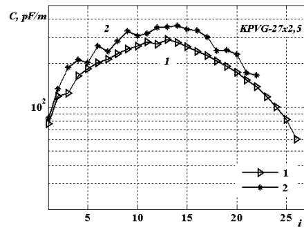
Рис. 9. Зависимости емкости отрезка кабеля КПВГ-27х2,5 от числа задействованных жил: 1 – расчетная; 2 – экспериментальная. Нумерация жил – из центра против часовой стрелки - наружу кабеля. Измеряется емкость i параллельно включенных жил относительно (27- i ) остальных
