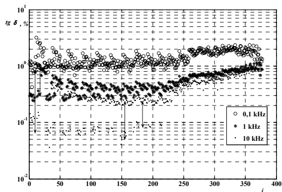
Рис. 10. Зависимости тангенса угла диэлектрических потерь отрезка кабеля КПВГ-27х2,5 от числа опытов: i меняется от 1 до 377. Отчетливо проявляется различие по \operatorname{tg} \delta на частоте 10 кГц
