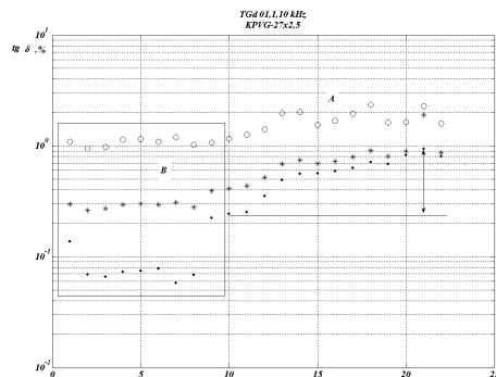
Рис. 3. Динамика изменений тангенса угла диэлектрических потерь от числа задействованных жил при измерении 27-жильного кабеля КПВГ
