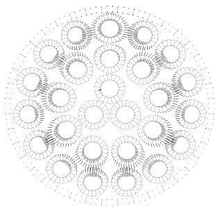
а) 13 потенциальных жил – против 14 нулевых жил
