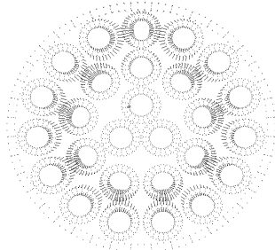
Рис. 8. То же, что и на рис. 6а, только 13 нулевых жил – против 14 потенциальных жил
