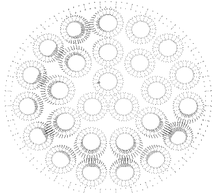
в) 17 потенциальных жил – против 14 нулевых жил
