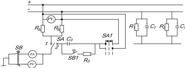
Рис. 2. Розрахункова схема для визначення омичного опору полюсів мережі відносно землі
