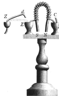
Рис. 5. В. Старджен (1783-1850) и конструкция его электромагнита
