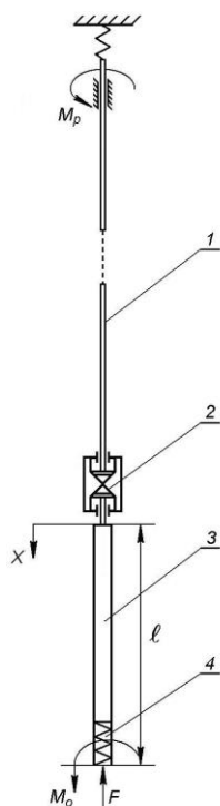
Рисунок 1 – Схема бурильної колони
