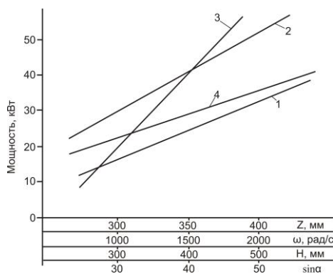
Рисунок 4 – Изменение потребляемой мощности при агломерации в зависимости от длины лопасти Z (1), угловой скорости перемешивания ω (2), высоты слоя материала H (3) и угла атаки ножей sin α (4)
