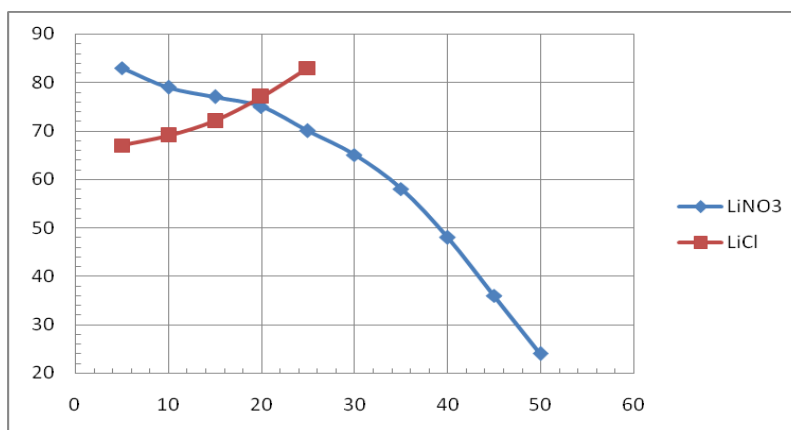
Рисунок 2 – Залежність світлопропускання модифікованих стекел від концентрації іонів литія
