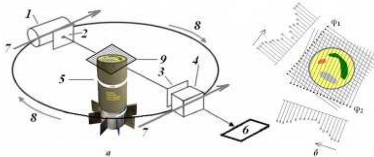
Рисунок 2 – Принцип рентгено-томографического сканирования боеприпаса
