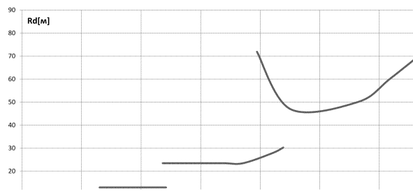
Рисунок 4 – Действительный радиус поворота (повышенная передача делителя, бетон)
