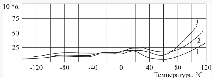
Рисунок 3 – Залежності \alpha_T = f(T) для вторинного поліетилену з різною кількістю геліфракції, %: 1 – 17; 2 – 34; 3 – 42
