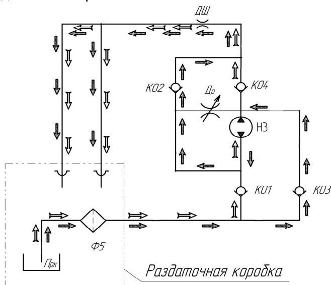
Рис. 1. Гидравлическая принципиальная схема смазки раздаточной коробки изделия БТР-4: Др - регулируемый дроссель; ДШ - дроссельная шайба; К01, К02, К03, К04 – обратные клапана; НЗ - нагнетательный насос; Прк – поддон картера раздаточной коробки; Ф5 – всасывающий фильтр раздаточной коробки; \Rightarrow движение масла на смазку раздаточной коробки при движении бронетранспортёра вперёд; \Rightarrow движение масла на смазку раздаточной коробки при движении бронетранспортёра задним ходом.
