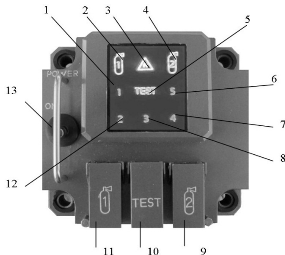
Рис. 4. Внешний вид блок-пульта ППО
