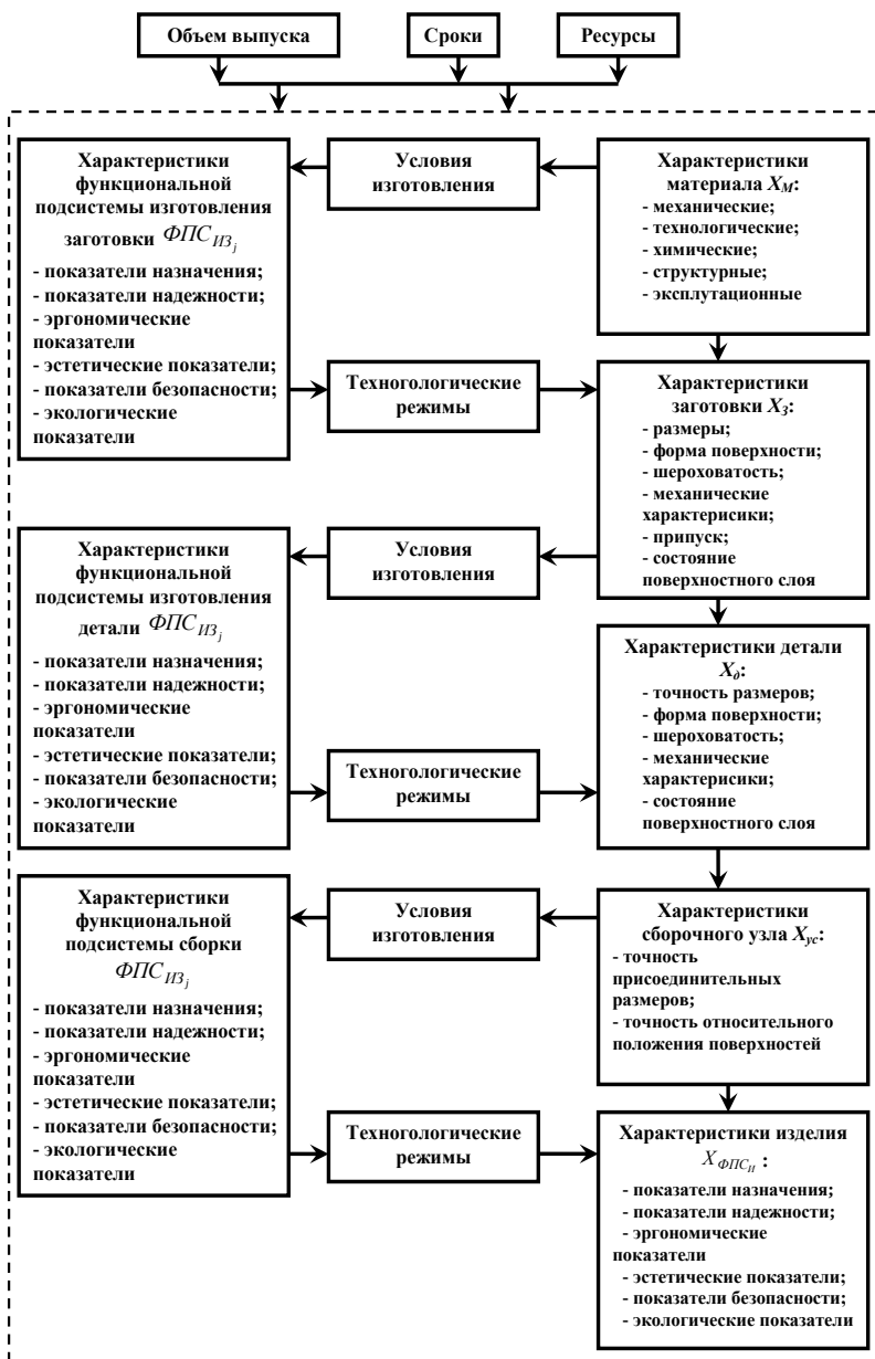
Рисунок 3 – Схема формирования характеристик изделия X_{ФПС_И}
