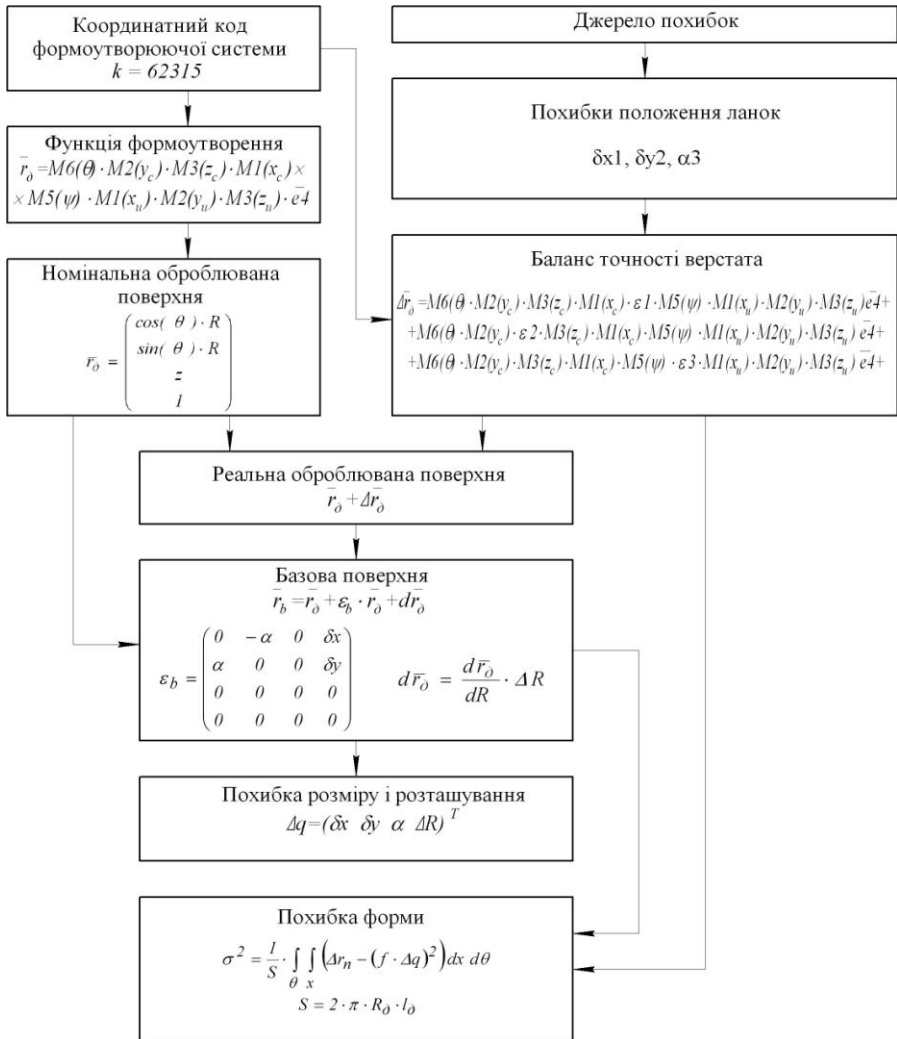
Рисунок 6 – Модель вихідної точності обробки голчасті циліндричної поверхні торцем бруска
