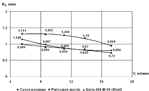
Рисунок 3 – Влияние СОТС на шероховатость поверхности при зенкеровании: (Р6М5; t = 0,5 мм; Титановый сплав BT1-0)
