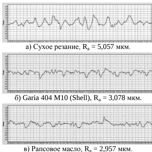
Рисунок 4 – Шероховатость зенкероманной поверхности втулок из стали 20
