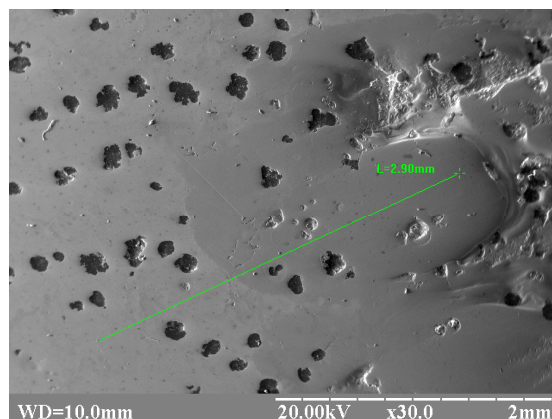
Рисунок 7 – Структура чавуну у дискретно зміцненій зоні; х30
