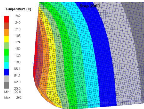
Рисунок 6 – Розподіл температурних полів у лезі інструменту із покриттям TiC
