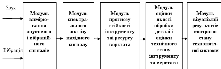
Рисунок 2 – Модулі, які складають програмну частину комплексу
