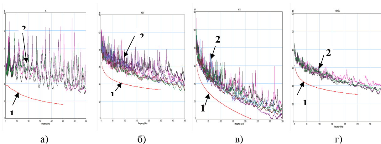
Рис. 3. Величина структурных возвратных потерь – SRL; а) дополнительные возвратные потери, обусловленные несовершенством конструкции кабеля (флуктуации диаметра токопроводящих жил, толщины изоляции, шагов скрутки пар); частотная зависимость для сетевого кабеля категории 5е: б) переходного затухания на ближнем конце сетевого кабеля; в) защищенности; г) суммарной мощности помех на ближнем конце при влиянии 3-х пар на одну в сетевом кабеле категории 5е
