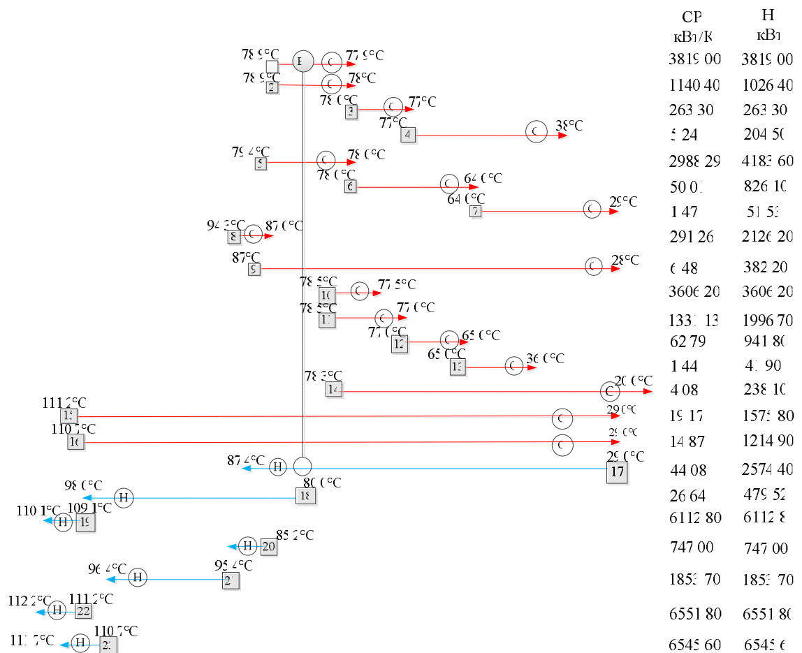
Рис. 2. Существующая система теплообмена на установке: 16 – горячие потоки; 17–23 – холодные потоки; CP– потоковая теплоемкость; ΔH – тепловые нагрузки для каждого потока
