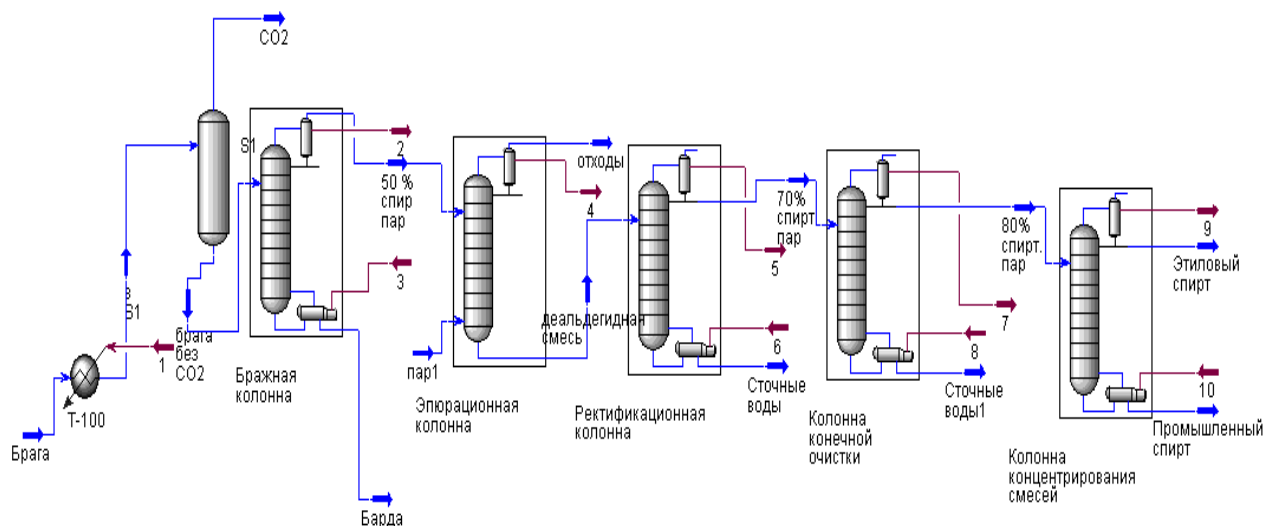
Рис. 4. Моделирование схемы в среде пакета UniSim Design
