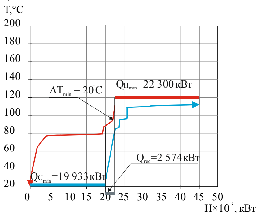
Рис. 3. Составные кривые существующего процесса: Q_{H_{\min}} - горячие утилиты; Q_{C_{\min}} - холодные утилиты, Q_{\text{rec}} - значение рекуперированной энергии
