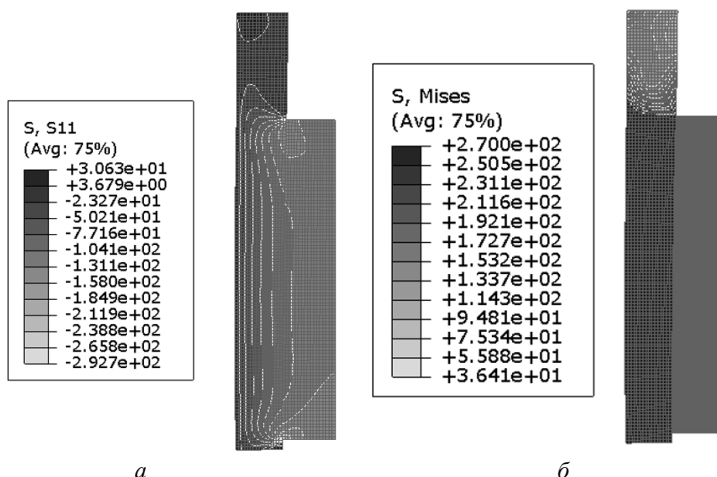
Рис. 3. Напряжения в биметаллическом соединении VT6-12X18N10T после нагрева: а – радиальные напряжения, МПа; б – напряжения Мизеса, МПа
