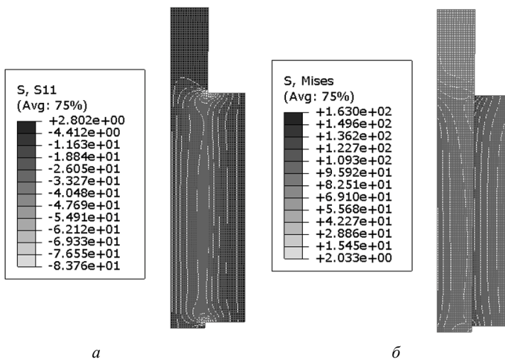
Рис. 2. Напряжения в биметаллическом соединении VT6-12X18N10T после запрессовки: а – радиальные напряжения, МПа; б – напряжения Мизеса, МПа
