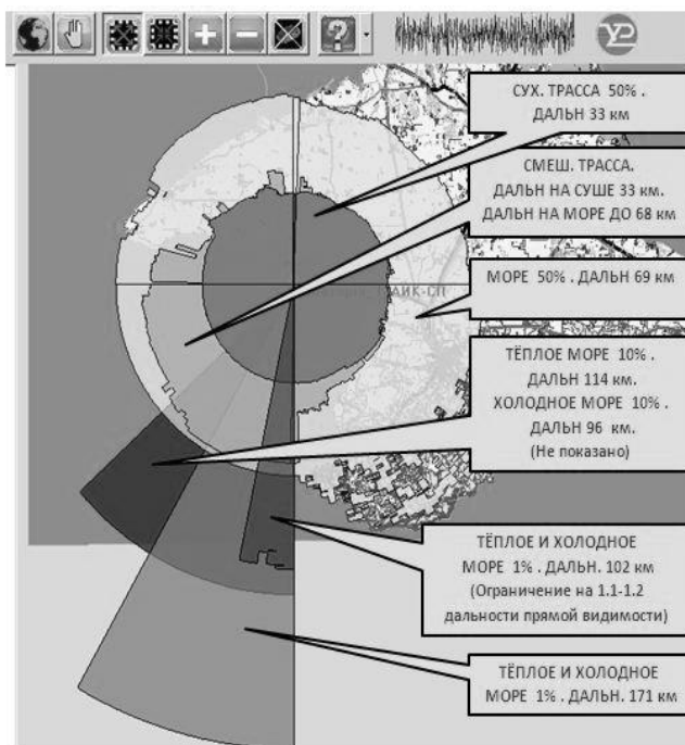
Рис. 2. Влияние различных факторов на величину зон радиодоступности
