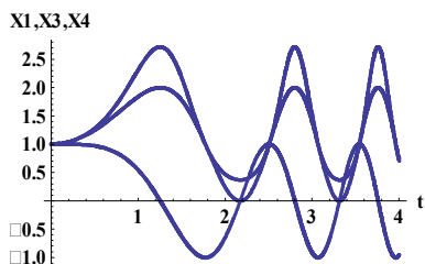
Рис. 1. Точные и численные решения по x_1(t), x_3(t), x_4(t)
