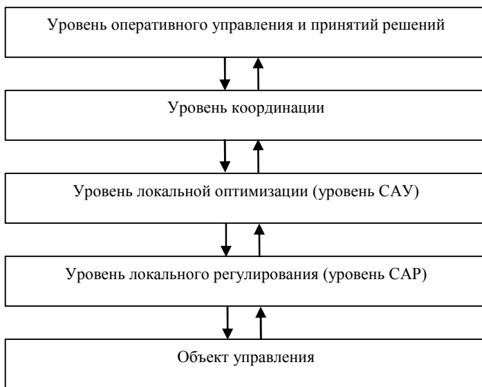
Рис. 1. Иерархическая структура системы управления
