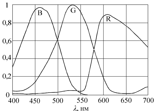
Рис. 1. Спектральные характеристики чувствительности ПЗС Samsung PL60 B – чувствительность синего канала; G – чувствительность зелёного канала; R – чувствительность красного канала
