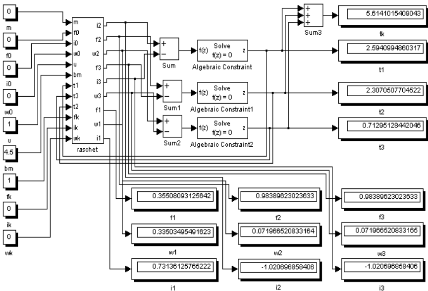
Рис. 1. Схема расчета параметров оптимального по быстродействию управления
