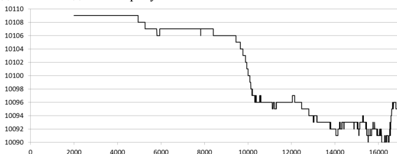
Рис. 4 Результат сглаживания медианным фильтром по 2000 отсчетам – не исключены погрешность квантования и систематическая погрешность
