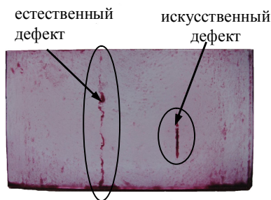
Рис. 5. Результат контроля.
