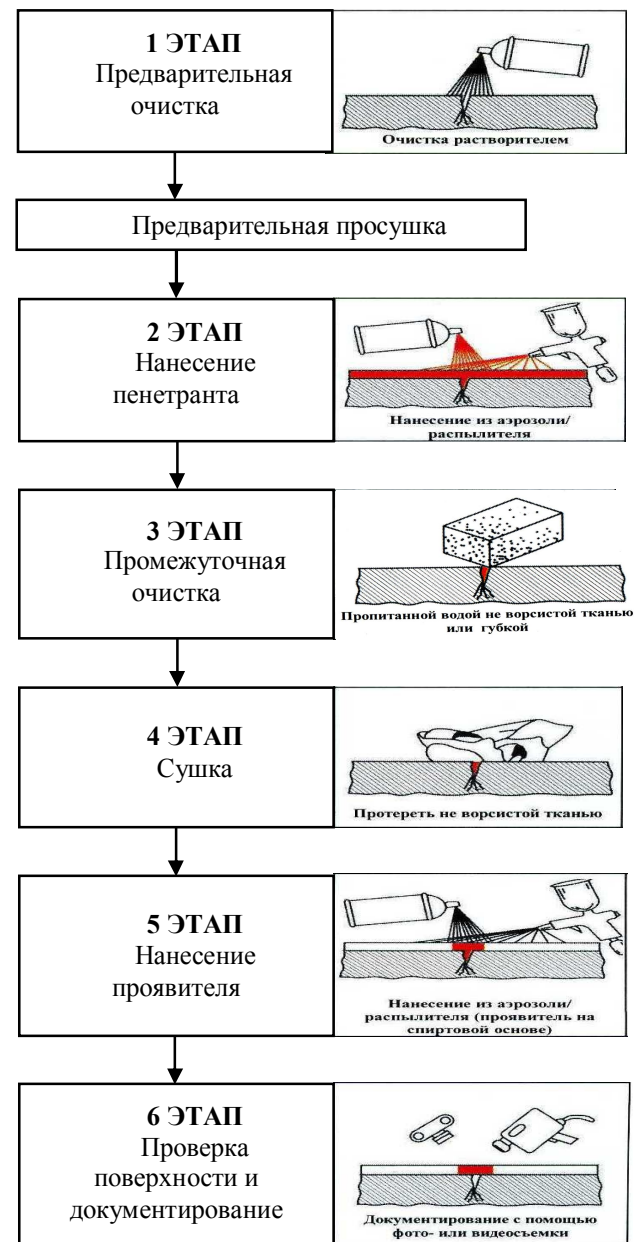
Рис. 1. Последовательность выполнения операций при капиллярном контроле детали цветным методом.
