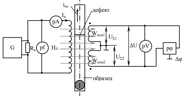
Рис. 1. Функциональная схема установки для определения дефектов в цилиндрических образцах.
