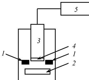
Рис. 3. Структурная схема радиоизотопной установки.
