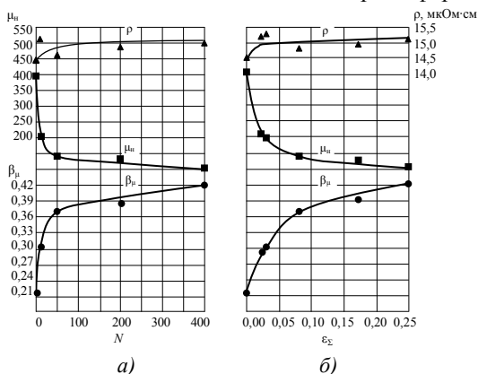
Рис. 2. Зависимость изменения удельного электрического сопротивления \rho начальной магнитной проницаемости \mu_n , значений вихретокового параметра \beta_\mu от числа циклов нагружения а) и величины накопленной пластической деформации б) образцов из стали 45.
