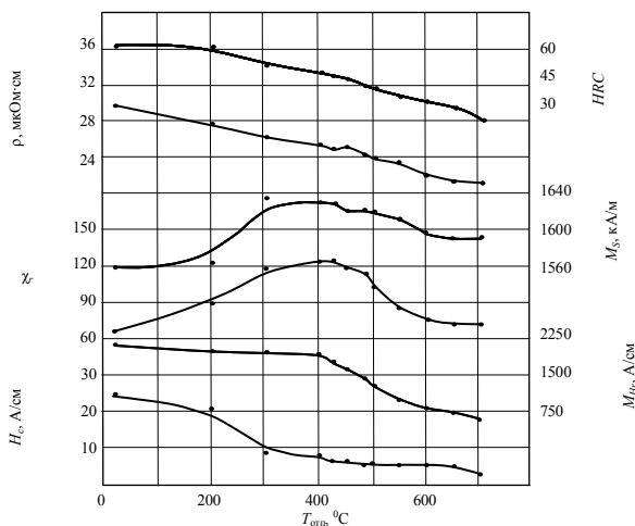
Рис. 1. Зависимости коэрцитивной силы H_c , релаксационных намагниченности M_{Hr} и магнитной восприимчивости \chi , намагниченности насыщения M_s , удельного электросопротивления \rho и твердости HRC из стали 45X1 от температуры отпуска T_{отп} .
