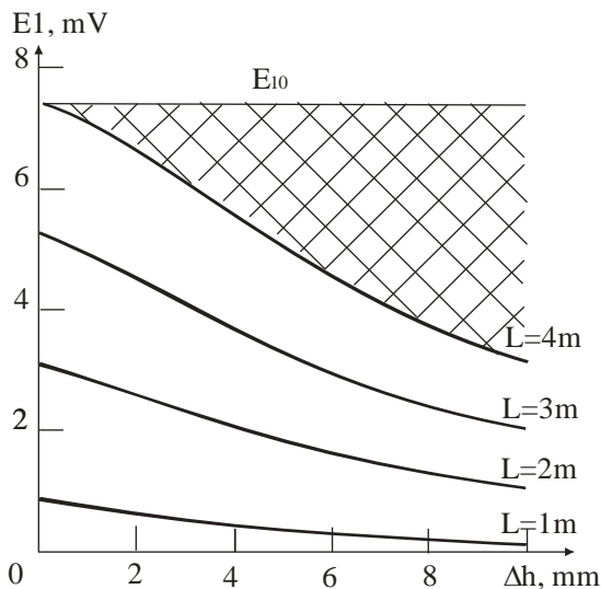
Рис. 3. Залежності амплітуди основного УЗС від зміни висоти нерівномірності поверхні рідинного середовища для різних рівнів
