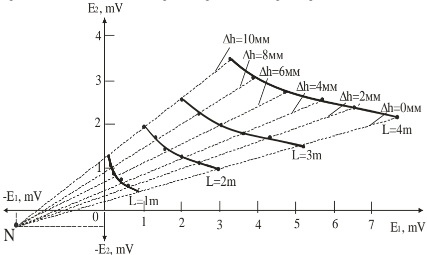
Рис. 5. Номограма залежності вторинного сигналу E_2 = f(E_1) для різних значень рівня та висоти нерівності рідинного середовища
