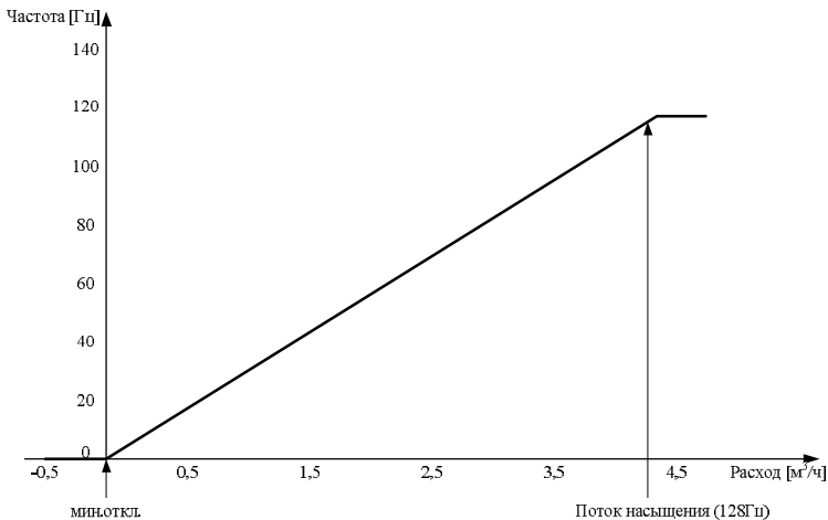
Рис. 1. Зависимость между частотой и расходом тепла.
