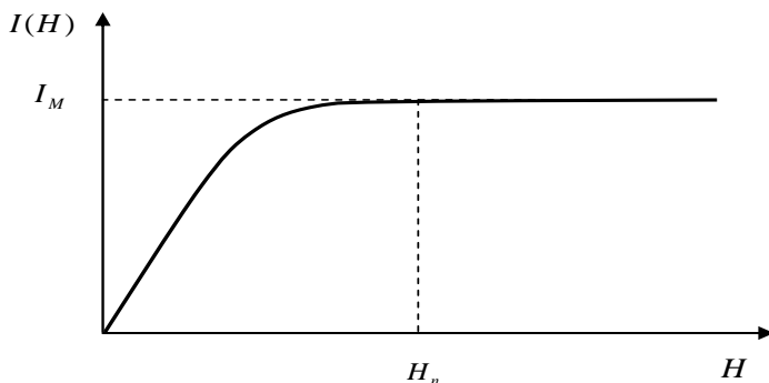
Рис.2. Зависимость намагниченности пульпы от напряженности магнитного поля
