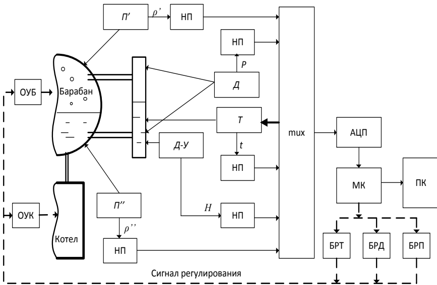
Рис. 5. Увеличенная структурная схема системы мониторинга уровня воды в барабане котла
