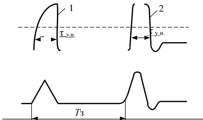
Рис. 4 – Форма электрического (1) и упругого (2) импульсов
