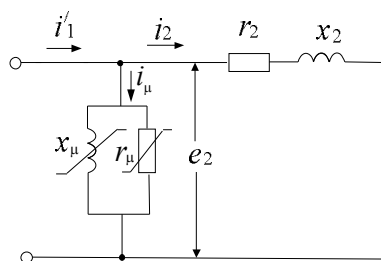
Рис. 1 – Схема замещения ТТ
