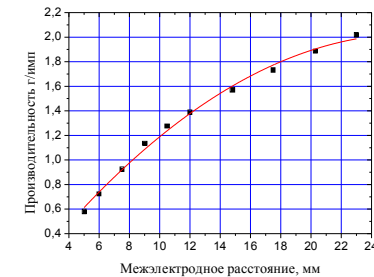
Рис.6 – Зависимость производительности резиновой крошки от межэлектродного расстояния
