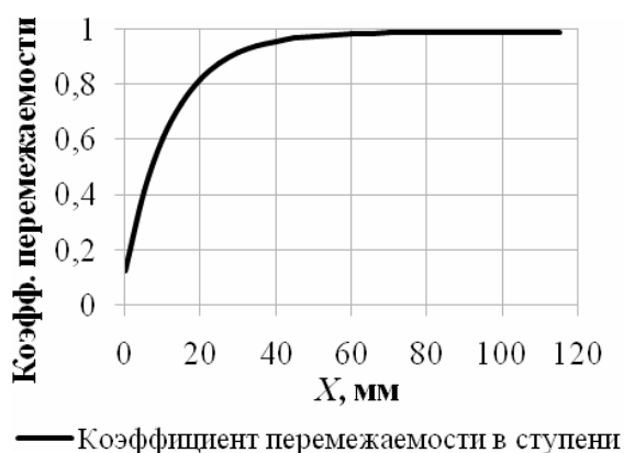
Рис. 2 – Розподілення коефіцієнта переважаємості по довжині турбінної ступені
