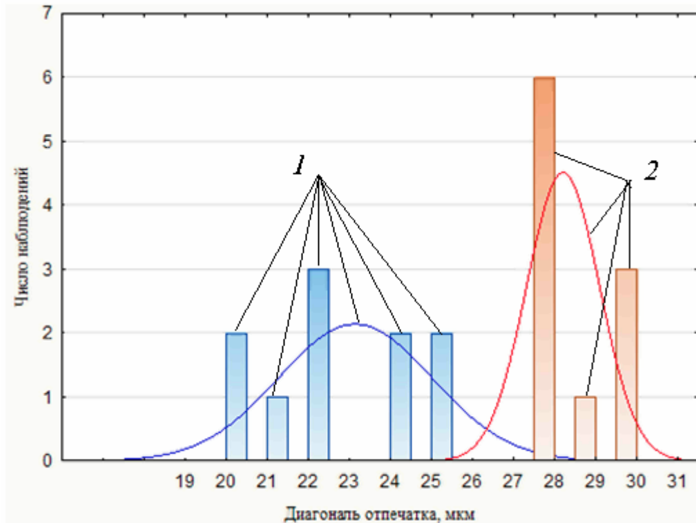
Рис. 4 – Гистограмма размеров отпечатков индентора на контрольном и обработанном паром образце при нагрузке 50 грамм: 1 – контрольный образец; 2 – образец, обработанный парокapelным потоком
