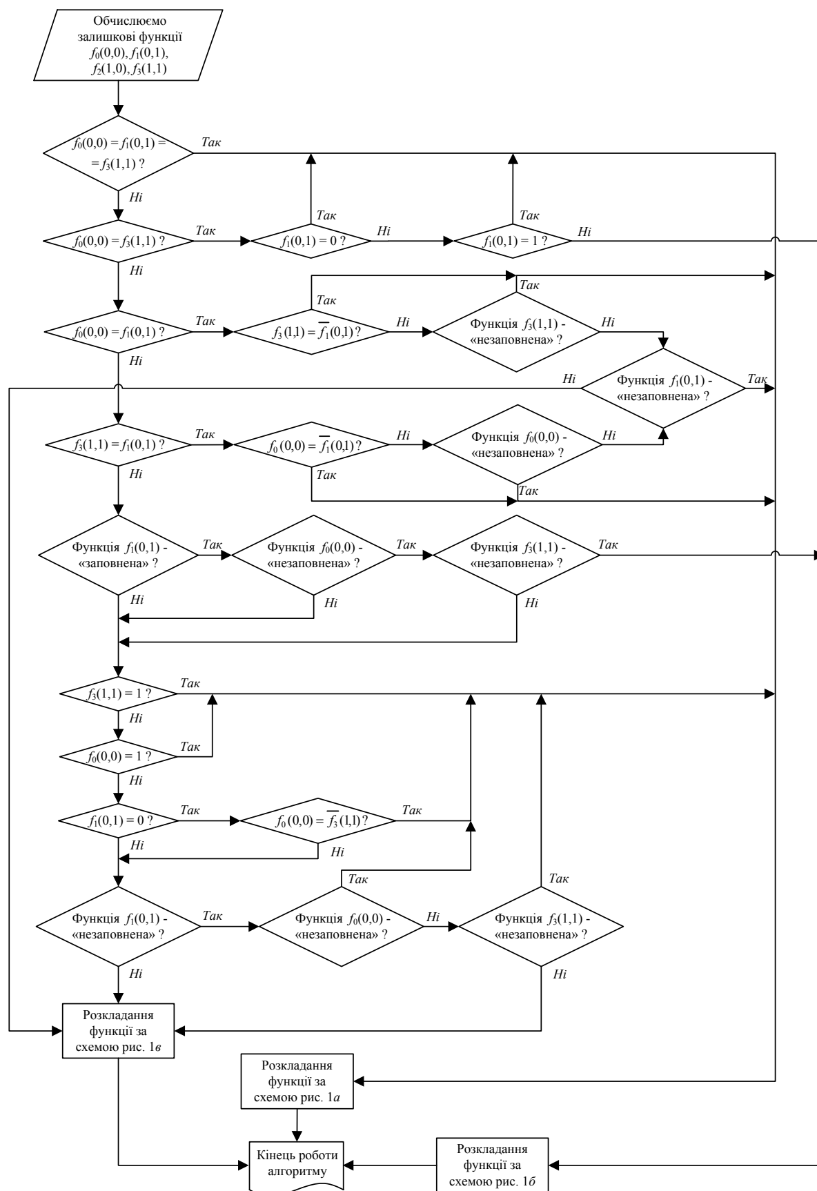
Рис. 3 –Алгоритм синтезу схем
