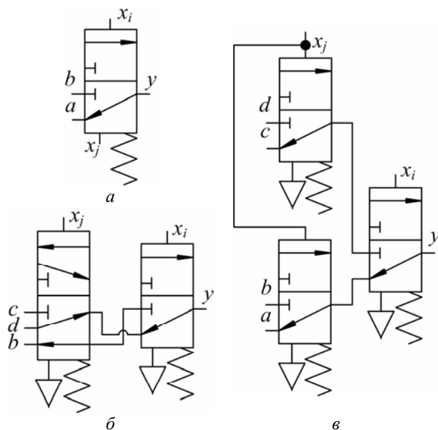
Рис. 1 – Схеми безроздільної декомпозиції функцій
