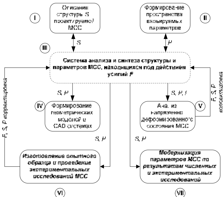
Рис.2. Структурная схема для организации процесса исследований машины для резки смеси
