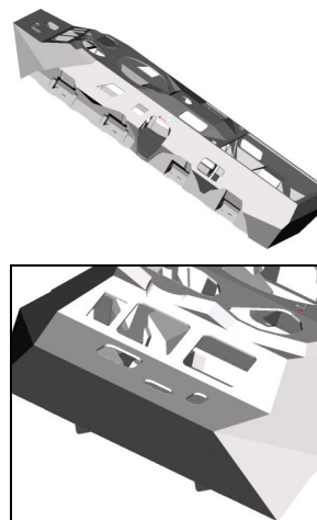
Рис. 5. Параметрическая модель корпуса БТР-94Б в среде Pro/ENGINEER
