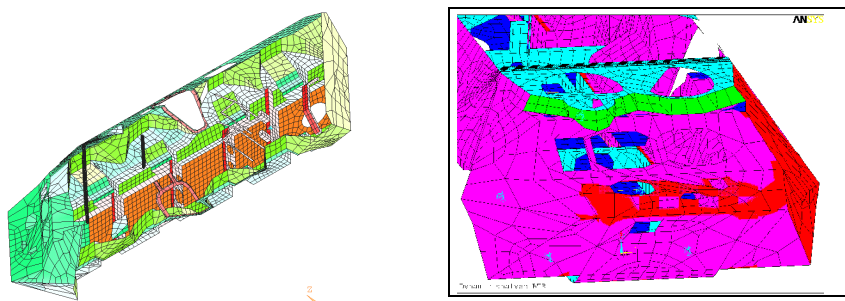
Рис. 6. Конечно-элементная модель корпуса БТР-94Б в среде ANSYS
