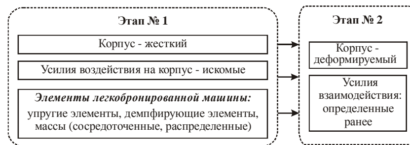
Рис. 2. Этапы решения задачи об исследовании динамических процессов в ходовой системе и напряженно-деформированного состояния корпуса ЛБМ
