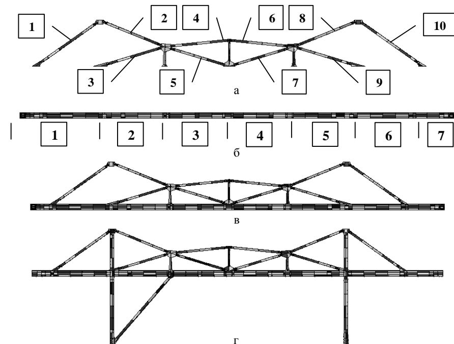
Рис. 2. Схема верхнего строения мостового перегружателя с номерами структурных элементов
