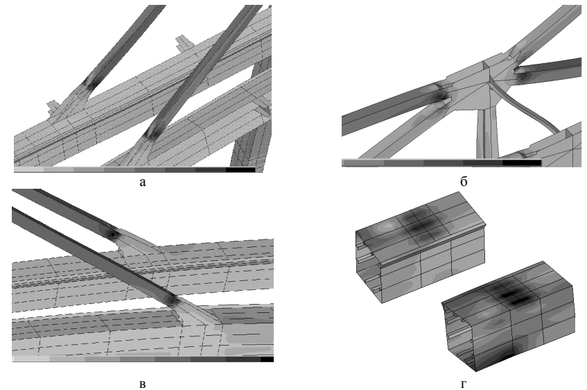
Рис. 3. Графическое представление эквивалентных напряжений (по Мизесу) в структурных элементах конструкции: а – ремонтная консоль; б – стойка; в – шарнирная опора; г – элемент секции балки
