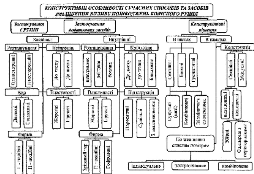
Рис. 29. Класифікація засобів з патентних джерел щодо зменшення впливу пошкоджень на динамічні якості машини
