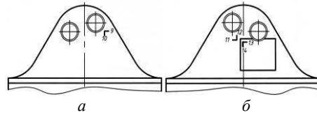
Рис. 4 – Схема установки тензорезисторов на стенках дебалансов: а – левая сторона, б – правая сторона
