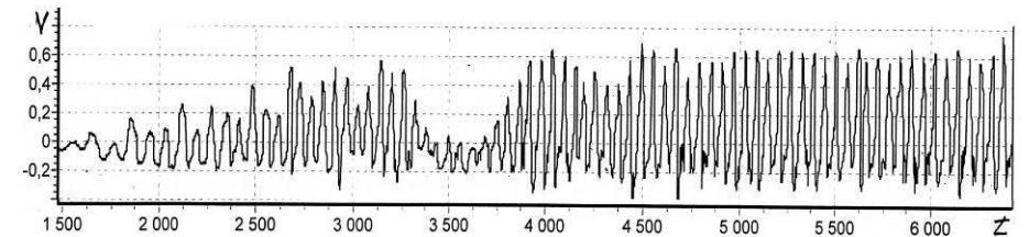
Рис. 9 – Осциллограмма напряжений (балка 3, точка 5, начало обработки, 2000 ед. \approx 1 с)
