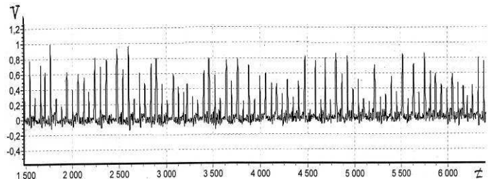
Рис. 6 – Осциллограмма напряжений (балка 1, точка 1, установившийся режим, 2000 ед. \approx 1 с)
