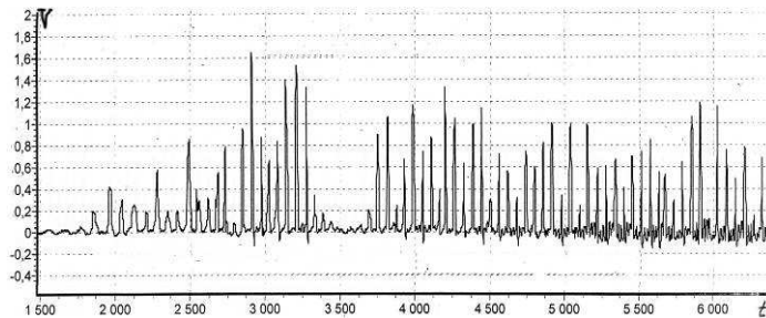
Рис. 5 – Осциллограмма напряжений (балка 1, точка 1, начало обработки, 2000 ед. \approx 1 с)
