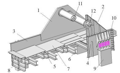
Рис. 2 – Общий вид опытного образца выбивной транспортирующей машины (показана часть модели)
