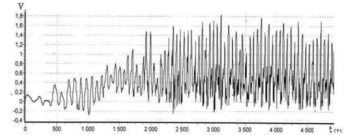
Рис. 7 – Осциллограмма напряжений (балка 2, точка 2, начало обработки, 2000 ед. \approx 1 с)
