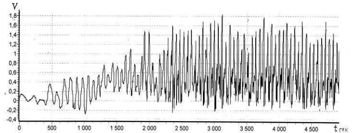
Рис. 8 – Осциллограмма напряжений (балка 2, точка 2, начало обработки, 2000 ед. \approx 1 с)
