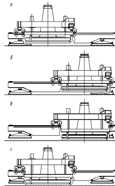
Рис. 8 – Цикл перешагивания отвалообразователя ОШС-4000/125
