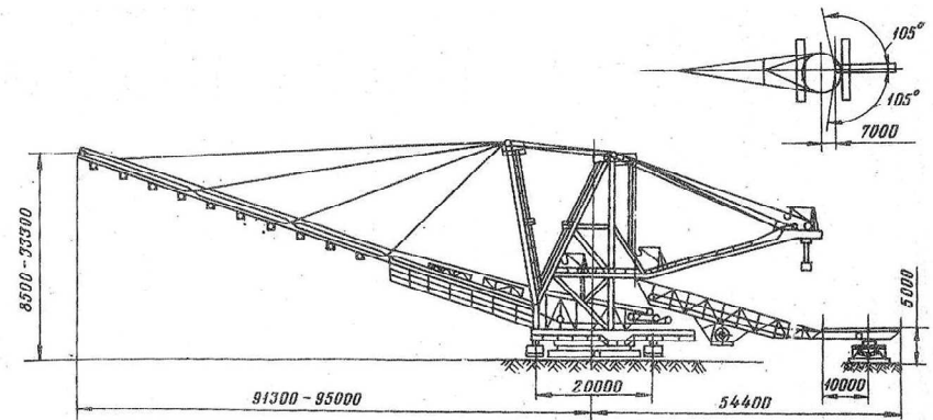
Рис. 3 – Конструктивная схема отвалообразователя ОШP-5000/95
